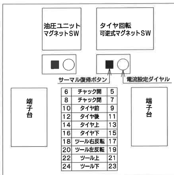
標準仕様コントロールボックスの内部
