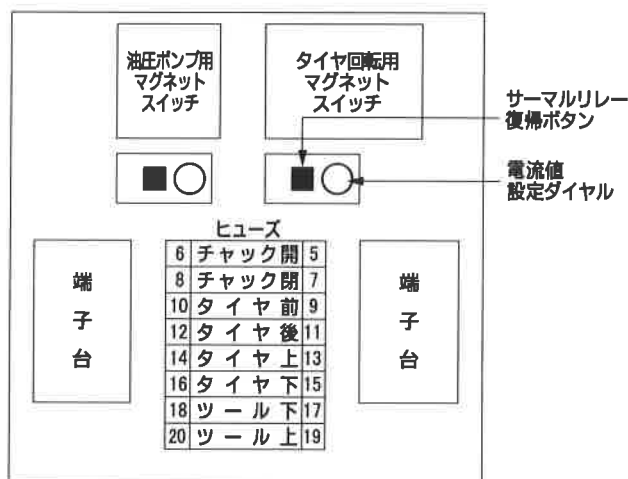
コントロールボックスの内部
