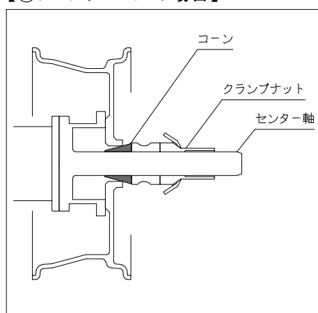
【②フロントコーンの場合】
