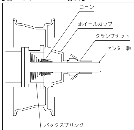
【①バックコーンの場合】
