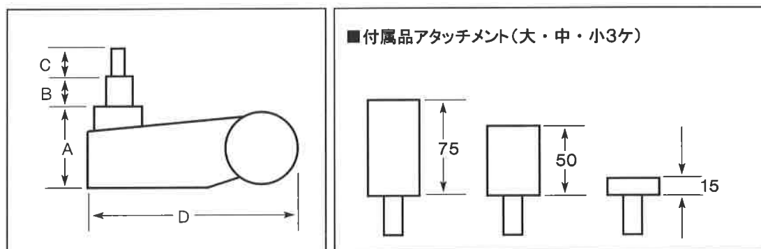
EXB-150W寸法図
