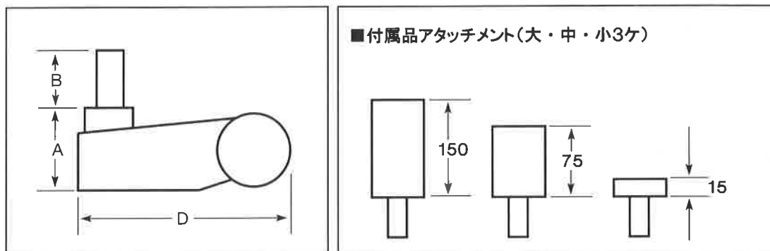
EXB-250・350寸法図
