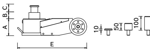
BAJ-120W spec3・BAJ-135W spec3・ BAJ-155W spec3 寸法図
