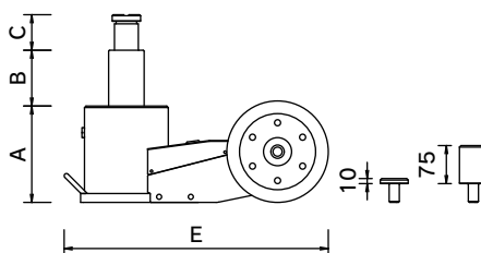
BAJ-300S spec3 寸法図
