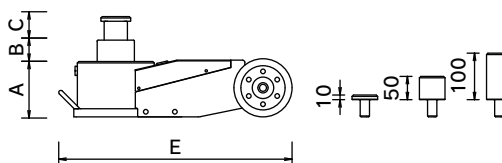
BAJ-120W・BAJ-135W・ BAJ-150W・BAJ-165W 寸法図
