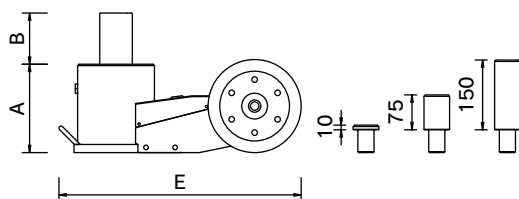
BAJ-120T 寸法図
