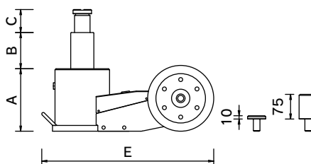
BAJ-300S 寸法図
