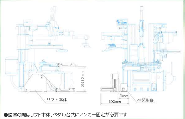
■ 設置寸法図
